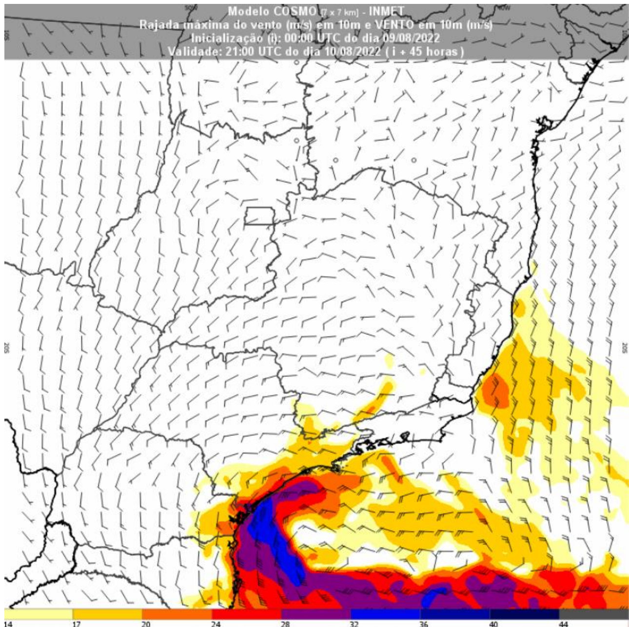
Figura 1 – Simulação do modelo COSMO/INMET com as rajadas de vento para os próximos dias. Unidade de medida em m/s.
