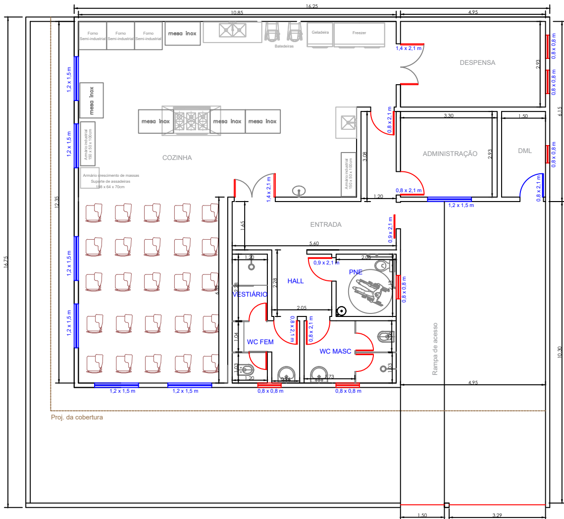
Planta Baixa – Cozinhamento
